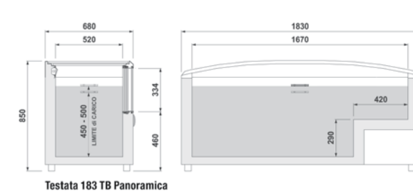
MODELLO 183 TESTATA PAN 1830 x 680 x 850
