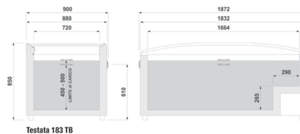
MODELLO 183 TESTATA 1830 x 880 x 850
