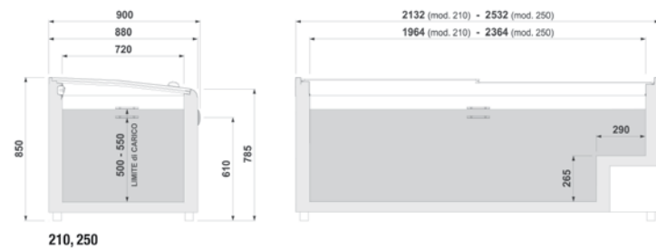
MODELLO 210 / 250 2130 x 880 x 850 / 2530 x 880 x 850
